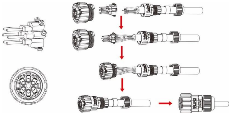
Figure 4.17 Connecteur DRM
