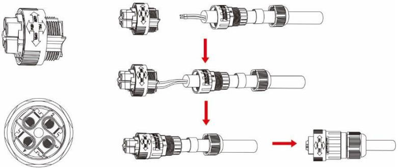
Figure 4.16 Connecteur CT
