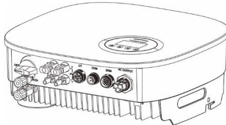
Figure 4.12 Raccordement des connecteurs DC à l'onduleur
