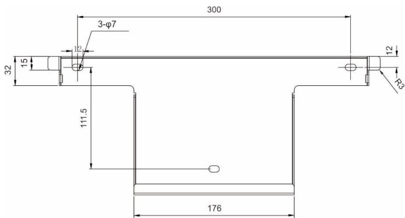
Figure 4.3 Montage mural de l'onduleur
