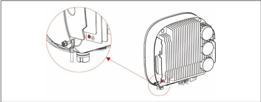
Figure 4.14 Raccordement du conducteur de mise à la terre externe
